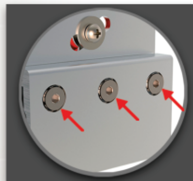
PRESIÓN UNIFORME A TRÁVES DE 3 TORNILLOS
