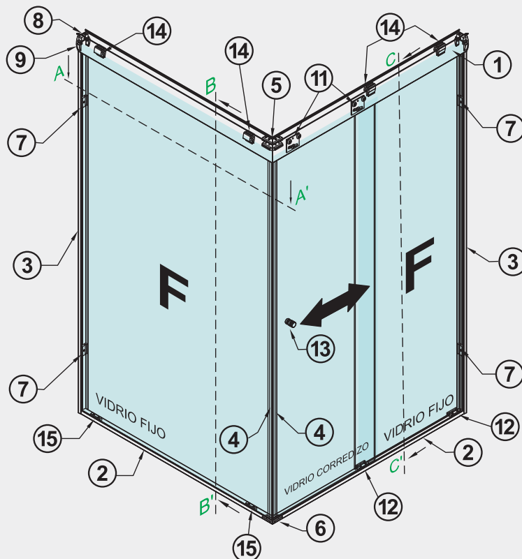
Cancel en Escuadra Fijo Exterior-Corredizo/Fijo Interior
