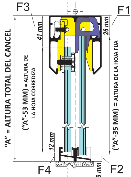
Carretilla Oculta (CON BARRENO)
