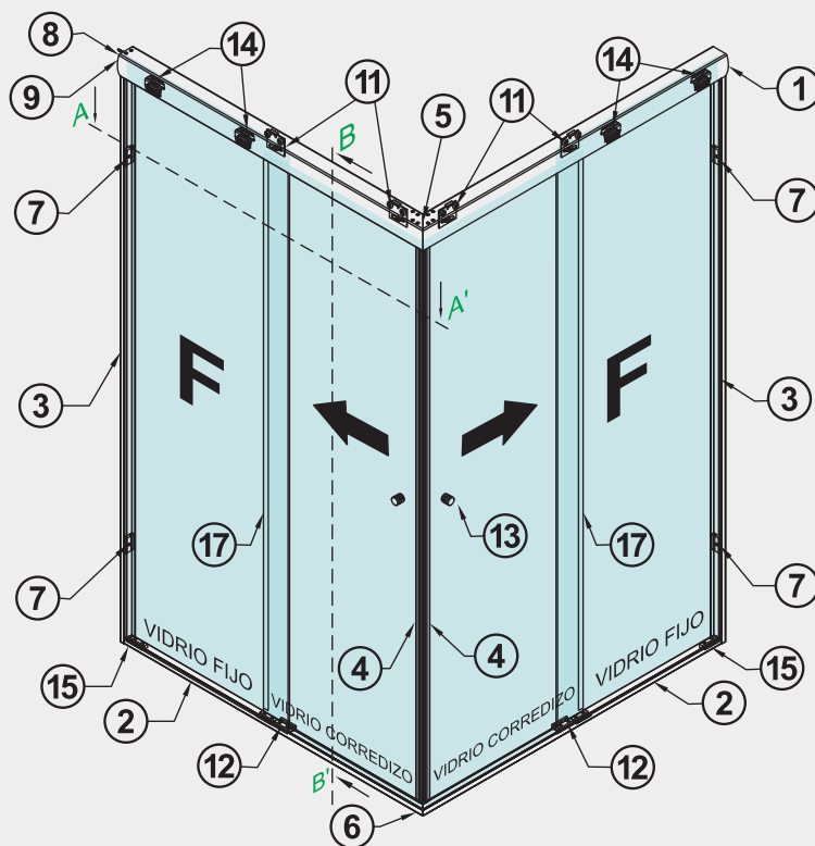
Cancel en Escuadra Fijo Exterior/Corredizo-Corredizo/Fijo Exterior
