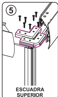
Cancel en Escuadra Fijo Exterior-Corredizo/Fijo Interior
